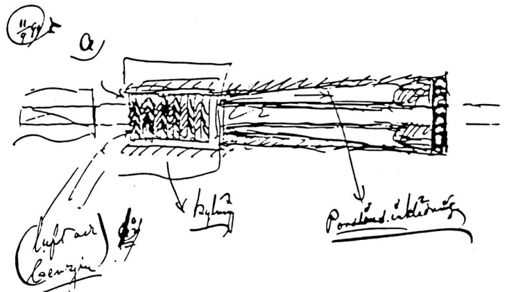
1899 års skiss över en gasturbin med flerstegs axialkompressor och porslinsklädd brännkammare.
